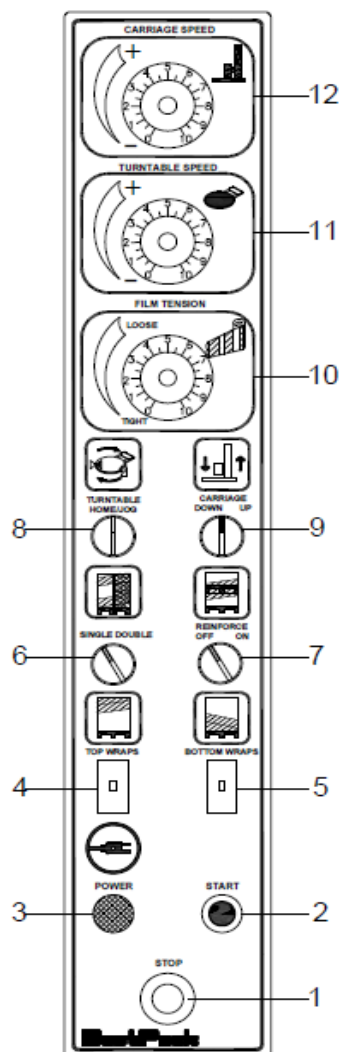
Bedieningspaneel SW-801
